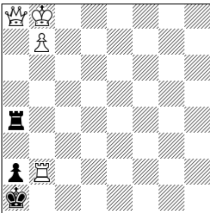
#3 1. ♖h2 1... ♜xa8 2. ba ♖(1) 1... ♜a7 2. ♖xa7(1) 1... ♜a6 2. ♖xa6(1) 1... ♜a5 2. ♖xa5(1) 1... ♜a3 2. ♖xa3(0.5) 1... ♖b1 2. ♖xa4(0.5)
