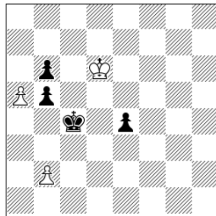
+ 1.a6 e3 2.a7 e2 3.a8 ♖(1) e1 ♖4. ♖d5+ ♖b4 5. ♖d3(2) ♖a1 6. ♖c3+ ♖a4 7.b3+(1) 5...c1 ♖ 6. ♖a3+ ♖c4 7.b3+(1)
