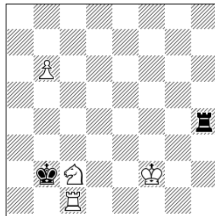
+ 1.b7 ♜h8 2. ♜h1(1) ♜b8 3. ♜a3(2) ♜xa3 4. ♜b1 ♜a4 5. ♜e3(1) ♜a5 6. ♜d4 ♜a6 7. ♜c5 ♜xb7 8. ♜a1#(1)
