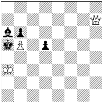
#3 1. ♖h1 1... ♜xb5 2. ♖d5(1.5) 1... ♜b7 2. ♖b1(1.5) 1...d4 2. ♖a8(2)
